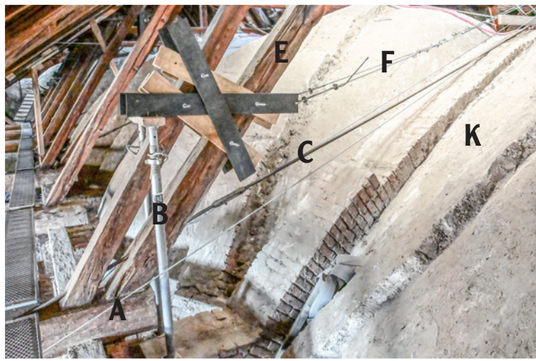
1. kép: A – kötőgerenda; B – menetes emelő; C – vas/kötőrúd; E – szelemengerenda; F – sodronykötél; K – boltozat
